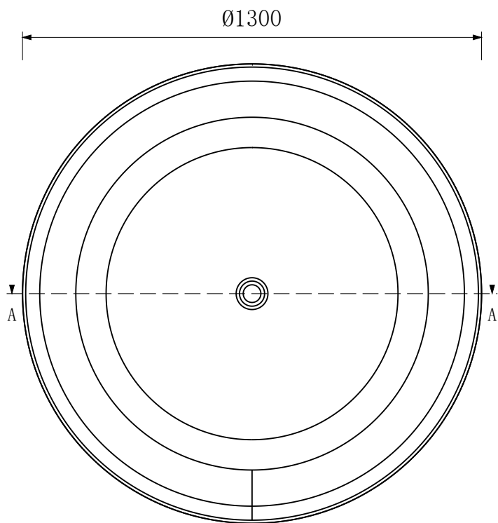
俯视图
