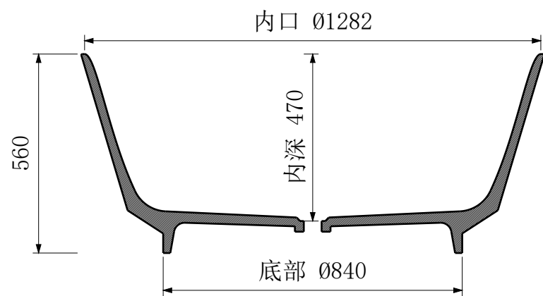
A-A 中心剖面
