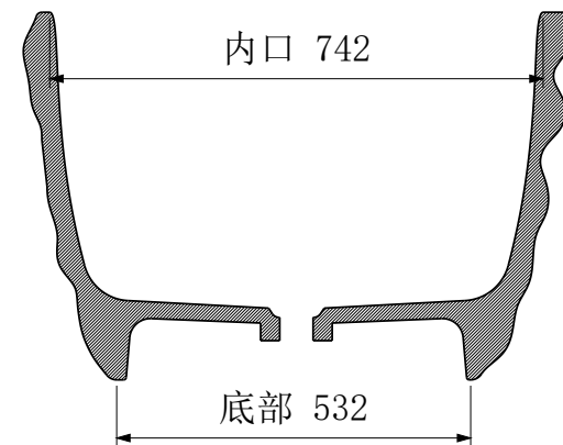
B-B 横向中心剖面
