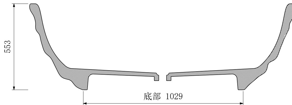
A-A 纵向中心剖面
