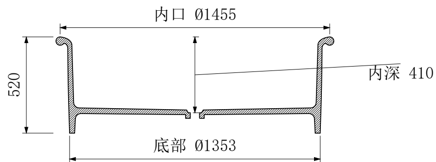
A-A 中心剖面
