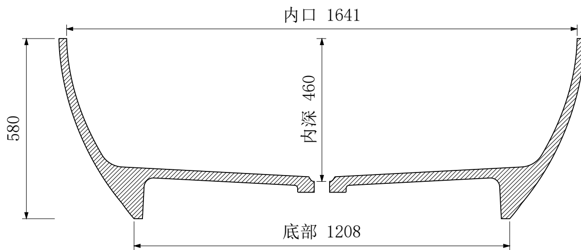
A-A 纵向中心剖面
