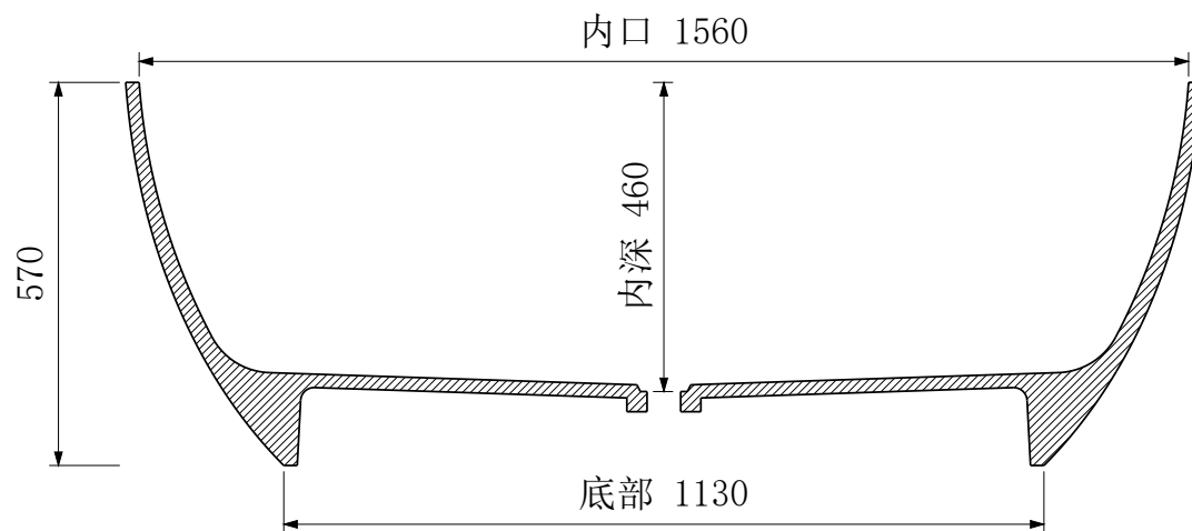
A-A 纵向中心剖面
