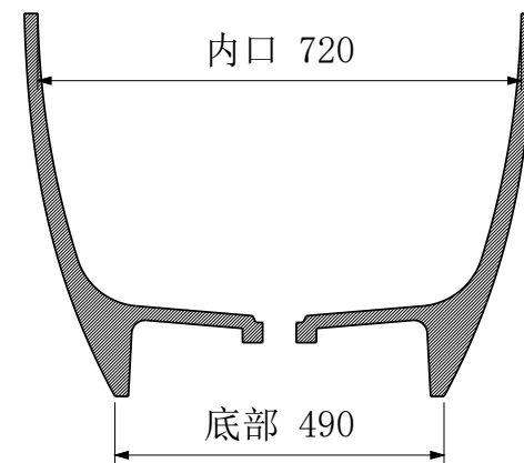
B-B 横向中心剖面
