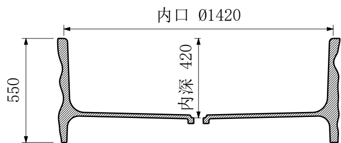
A-A 中心剖面
