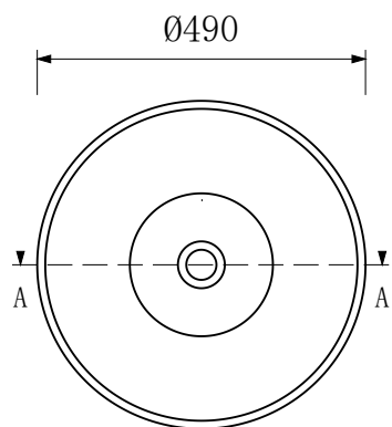
俯视图
