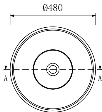
俯视图
