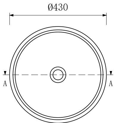
俯视图
