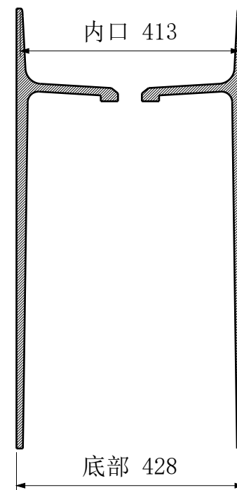
B-B 横向中心剖面
