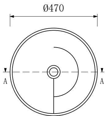
俯视图
