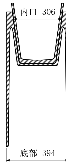
B-B 横向中心剖面
