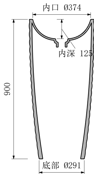
A-A 中心剖面
