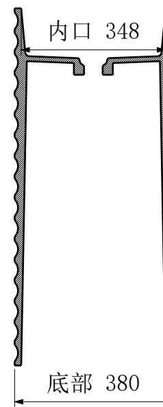
B-B 横向中心剖面
