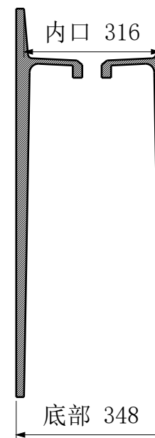
B-B 横向中心剖面
