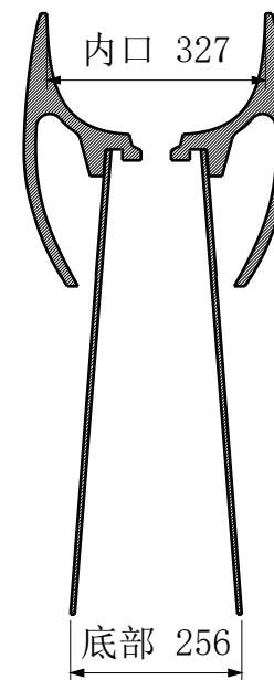
B-B 横向中心剖面
