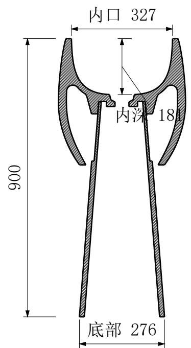
A-A 纵向中心剖面
