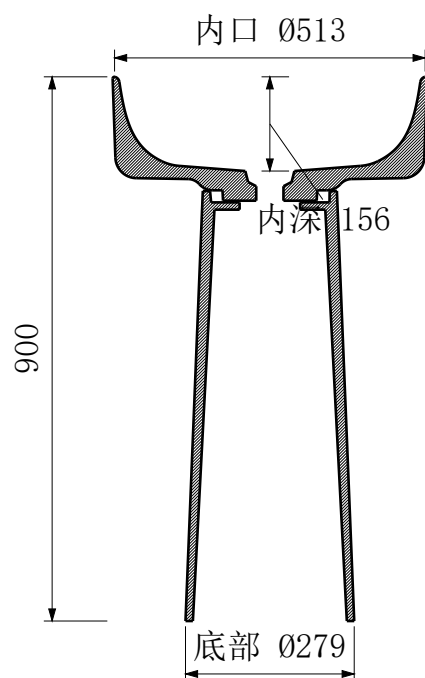
A-A 中心剖面
