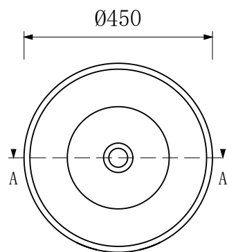
俯视图
