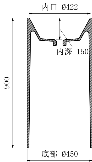
A-A 中心剖面
