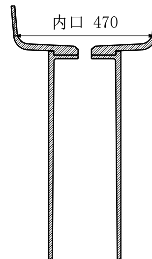
B-B 横向中心剖面
