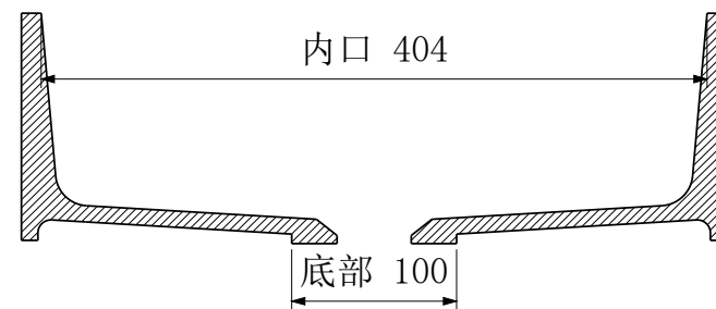
B-B 横向中心剖面
