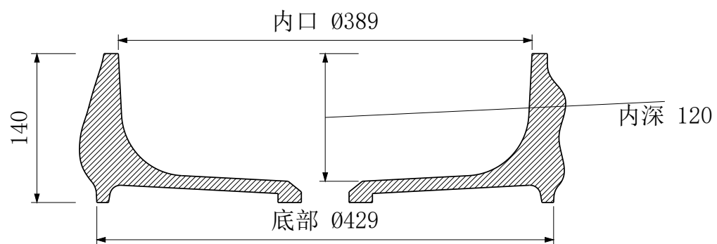
A-A 中心剖面
