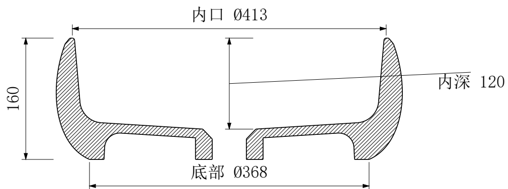
A-A 中心剖面
