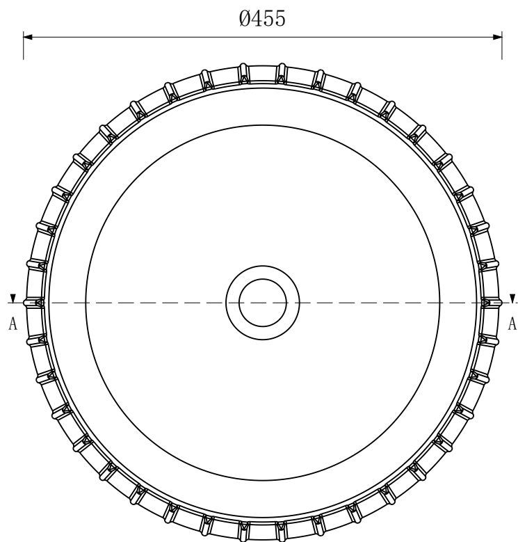
俯视图
