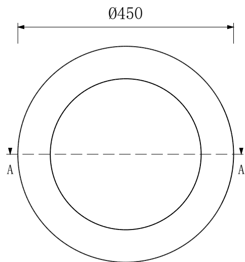
俯视图
