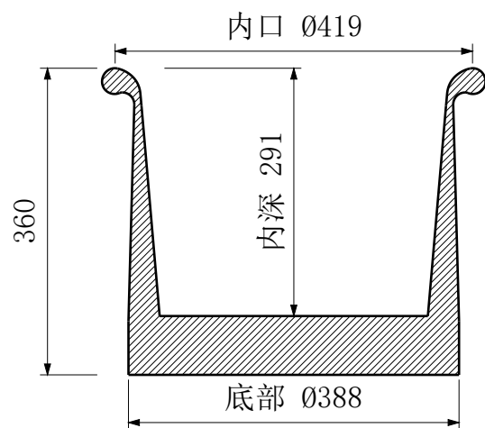
A-A 中心剖面
