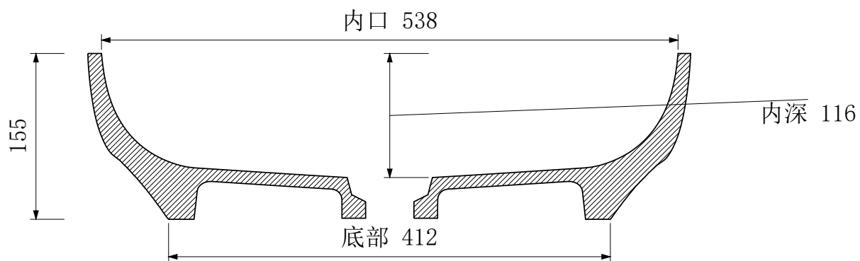
A-A 纵向中心剖面
