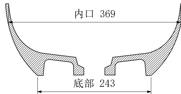
B-B 横向中心剖面
