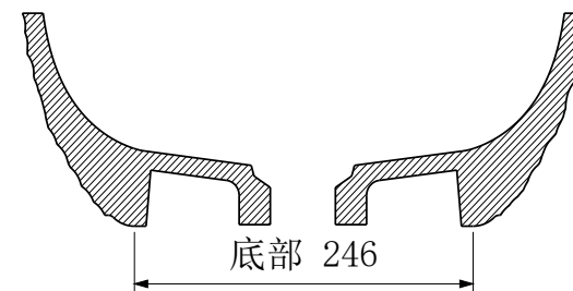
B-B 横向中心剖面
