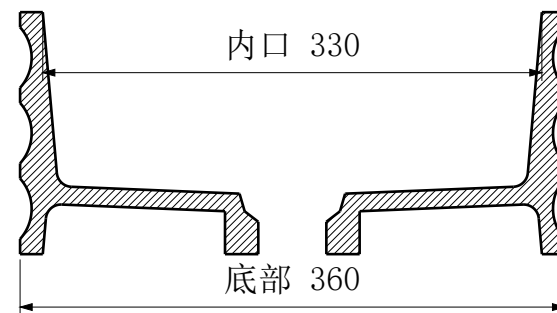
B-B 横向中心剖面
