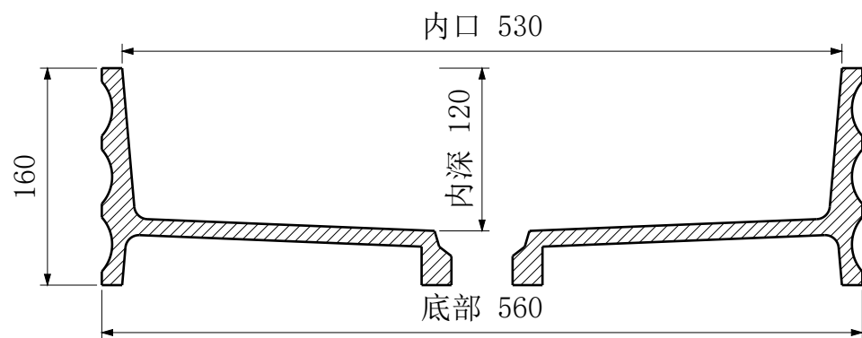
A-A 纵向中心剖面
