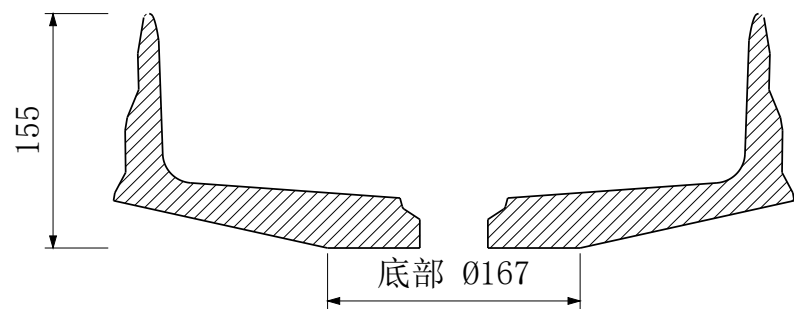
A-A 中心剖面
