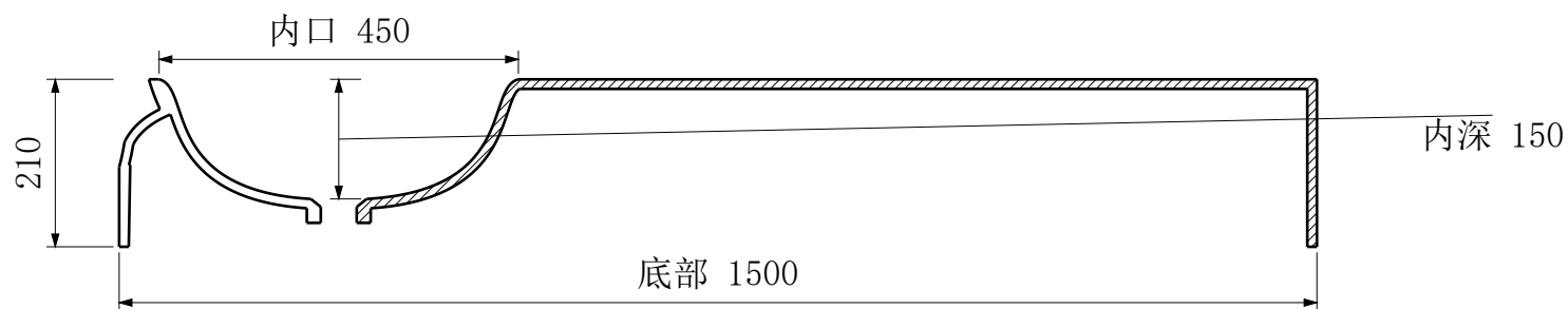
A-A 纵向中心剖面
