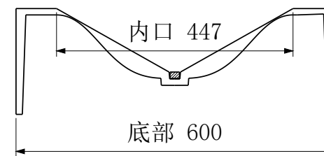
B-B 横向中心剖面
