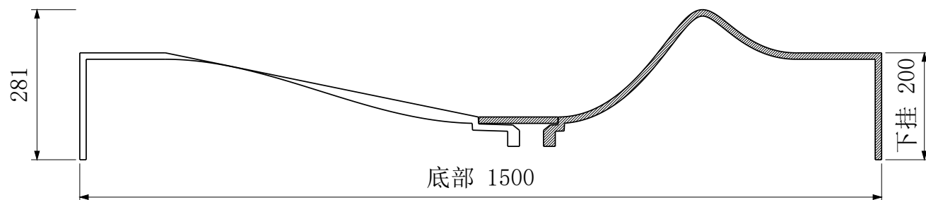
A-A 纵向中心剖面
