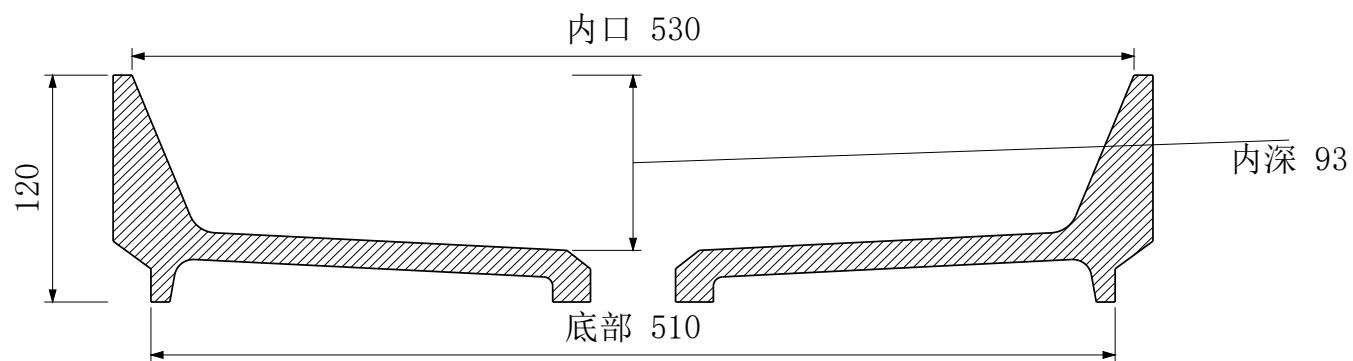
A-A 纵向中心剖面
