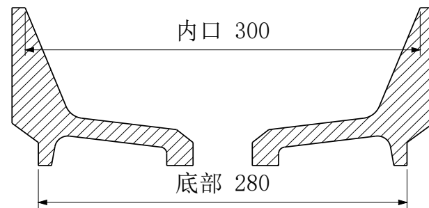
B-B 横向中心剖面
