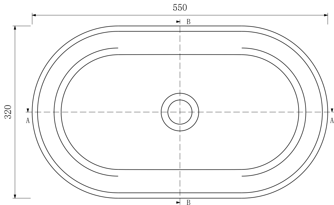
俯视图
