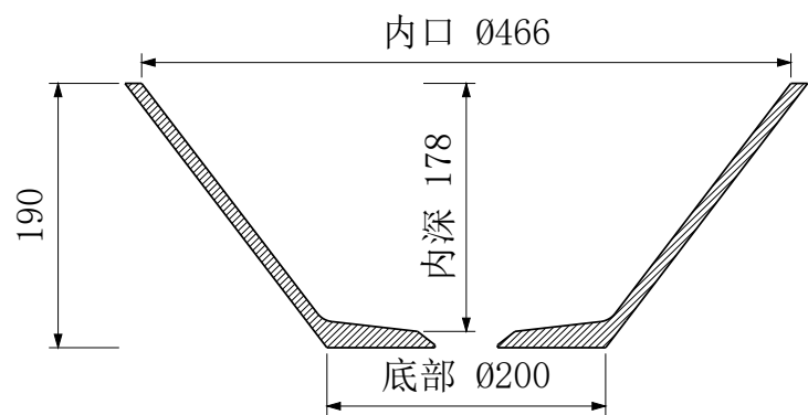
A-A 中心剖面
