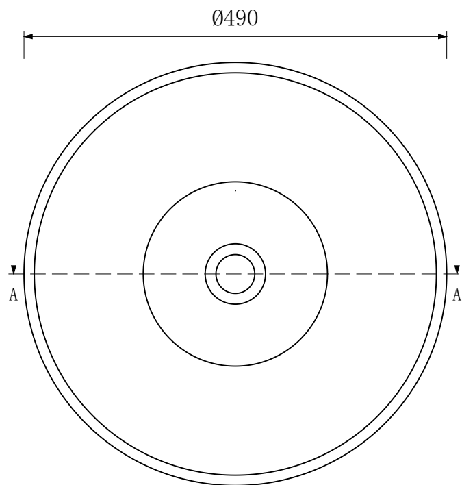
俯视图
