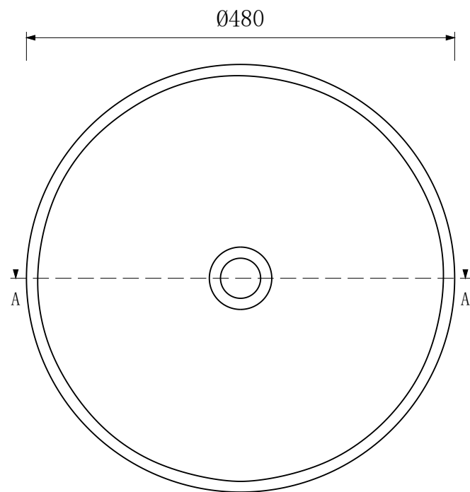
俯视图
