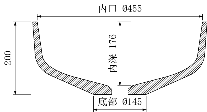
A-A 中心剖面
