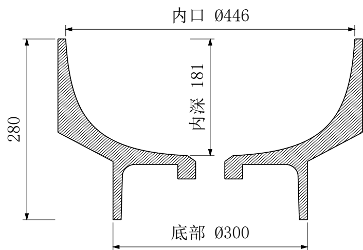
A-A 中心剖面
