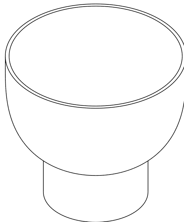
正等测线框 1:5
