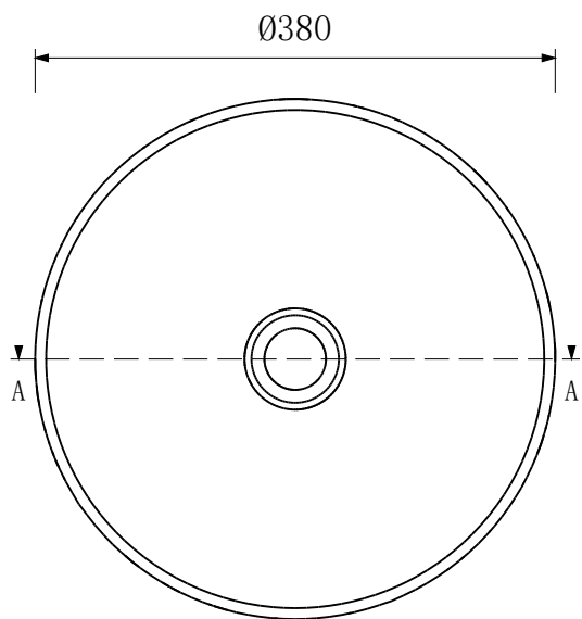
俯视图
