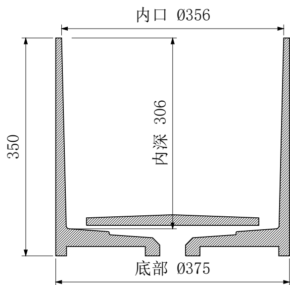
A-A 中心剖面
